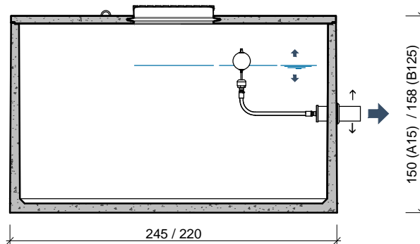
DOORSNEDE COUPE
