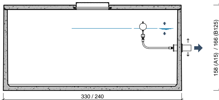
DOORSNEDE COUPE
