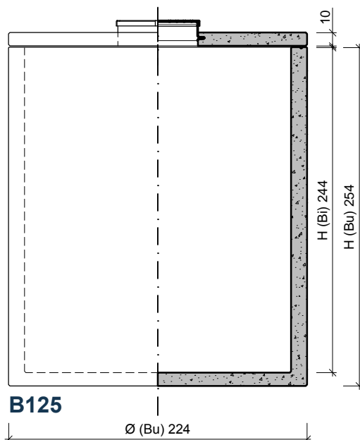
VOORAANZICHT / DOORSNEDE VUE FRONTALE / COUPE
