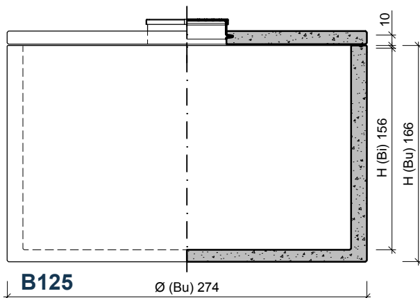
VOORAANZICHT / DOORSNEDE VUE FRONTALE / COUPE
