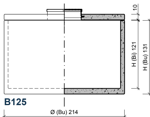
VOORAANZICHT / DOORSNEDE VUE FRONTALE / COUPE
