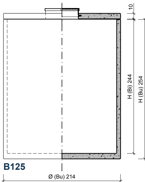
VOORAANZICHT / DOORSNEDE VUE FRONTALE / COUPE
