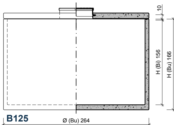
VOORAANZICHT / DOORSNEDE VUE FRONTALE / COUPE
