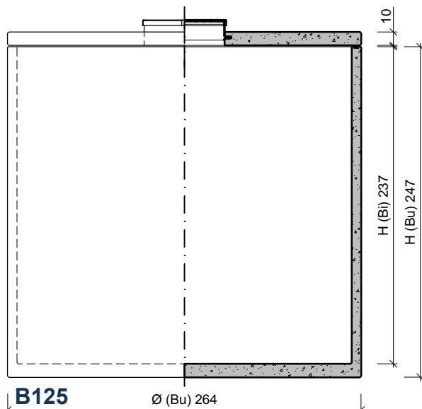
VOORAANZICHT / DOORSNEDE VUE FRONTALE / COUPE
