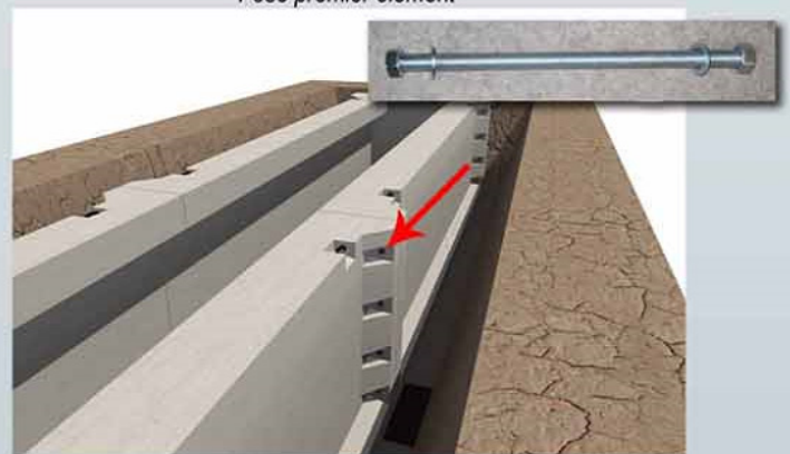
Plaatsen tweede element en vastschroeven betonnen elementen Pose deuxième élément et assemblage par boulonnage
