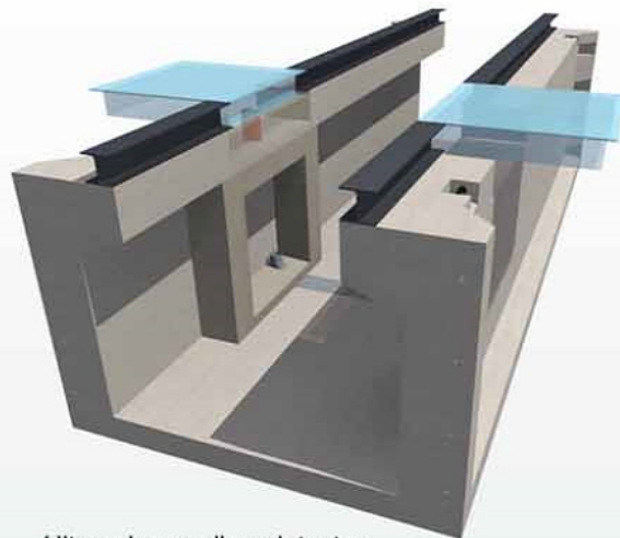
Uitsparing spelingsdetector Pré-équipement pour réception du cadre des plaques à jeux
