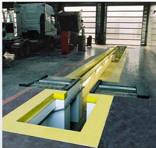
PUT VOOR REMTESTBANK
