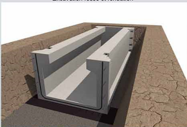
Plaatsen eindplaat Pose plaque d'embout
