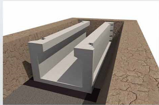
Plaatsen eerste element Pose premier élément
