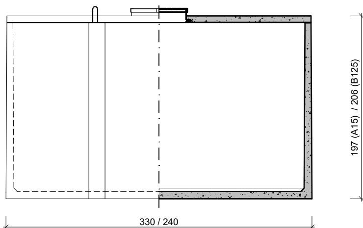
VOORAANZICHT / DOORSNEDE VUE FRONTALE / COUPE
