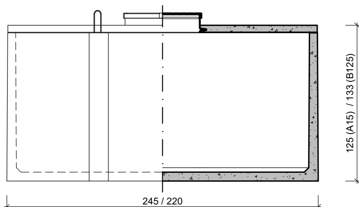
VOORAANZICHT / DOORSNEDE VUE FRONTALE / COUPE
