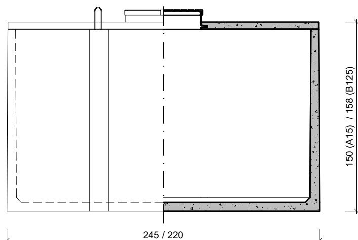
VOORAANZICHT / DOORSNEDE VUE FRONTALE / COUPE
