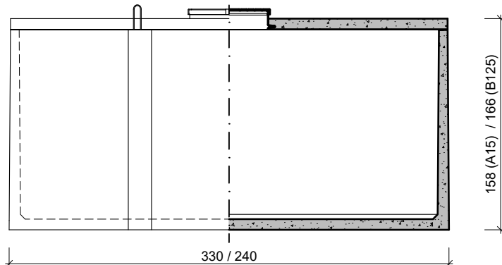
VOORAANZICHT / DOORSNEDE VUE FRONTALE / COUPE
