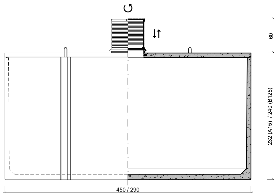
VOORAANZICHT / DOORSNEDE VUE FRONTALE / COUPE
