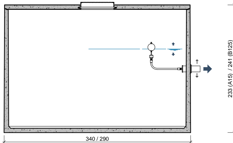
DOORSNEDE COUPE
