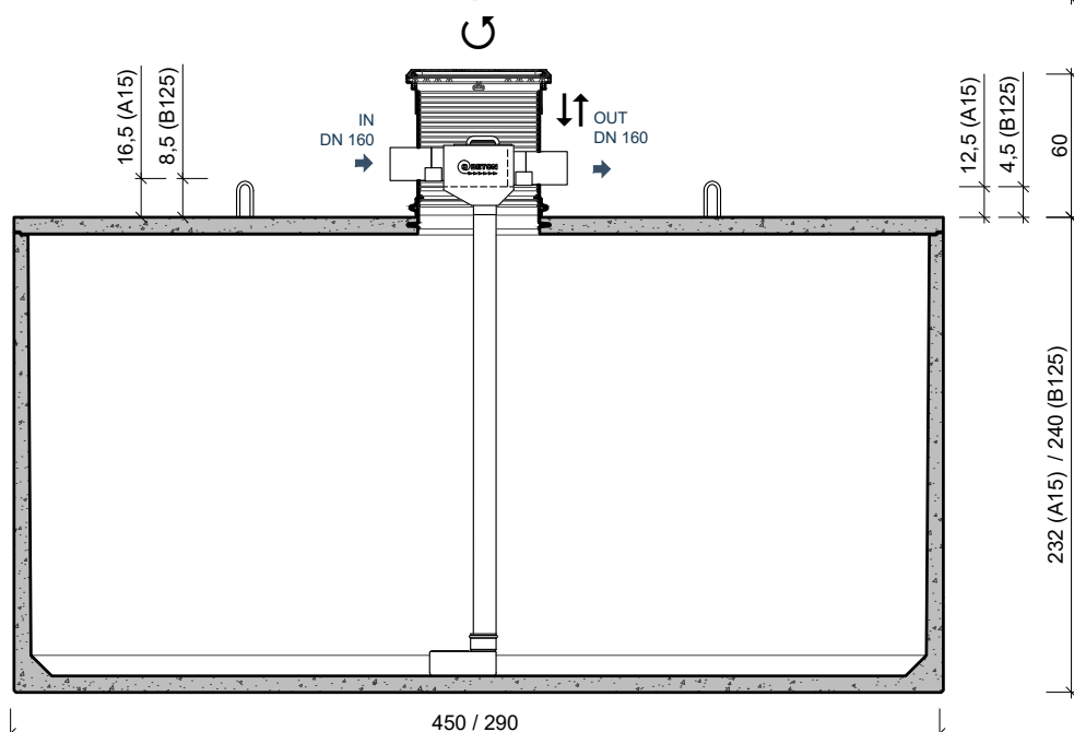
DOORSNEDE COUPE
