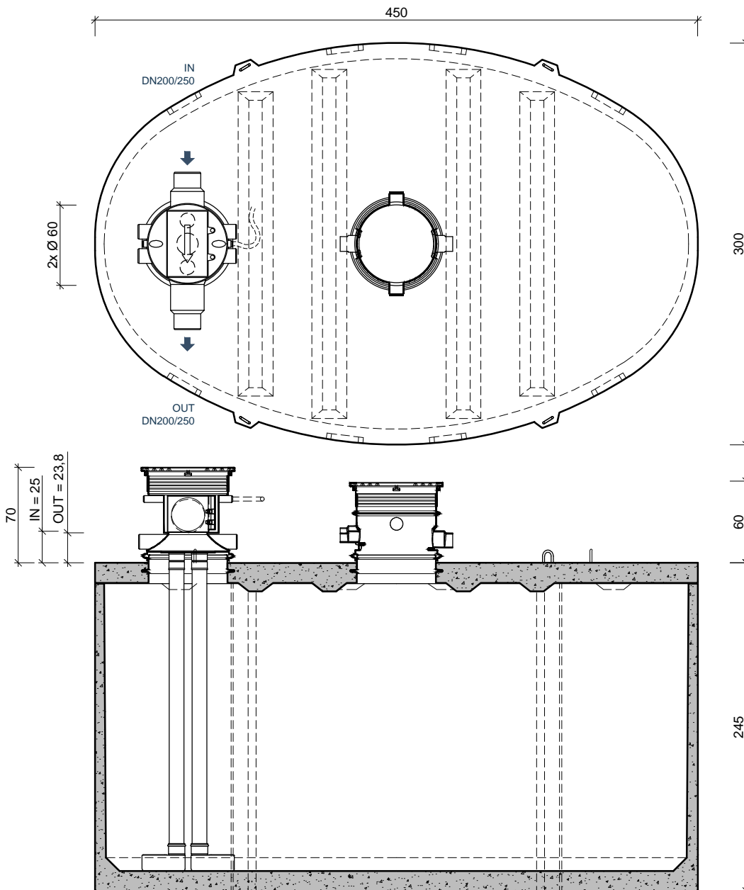
BOVENAANZICHT VUE DE DESSUS
