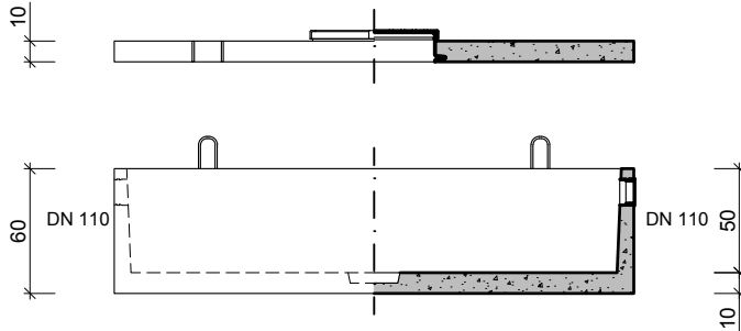
VOORAANZICHT / DOORSNEDE VUE FRONTALE / COUPE
