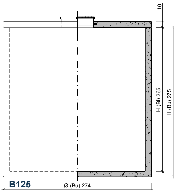
VOORAANZICHT / DOORSNEDE VUE FRONTALE / COUPE
