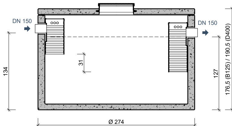
DOORSNEDE COUPE
