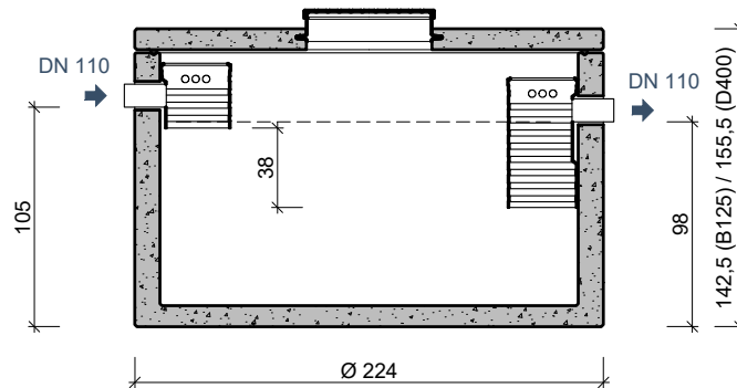
DOORSNEDE COUPE
