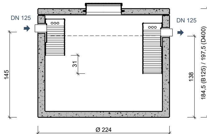
DOORSNEDE COUPE
