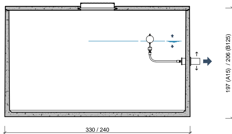
DOORSNEDE COUPE
