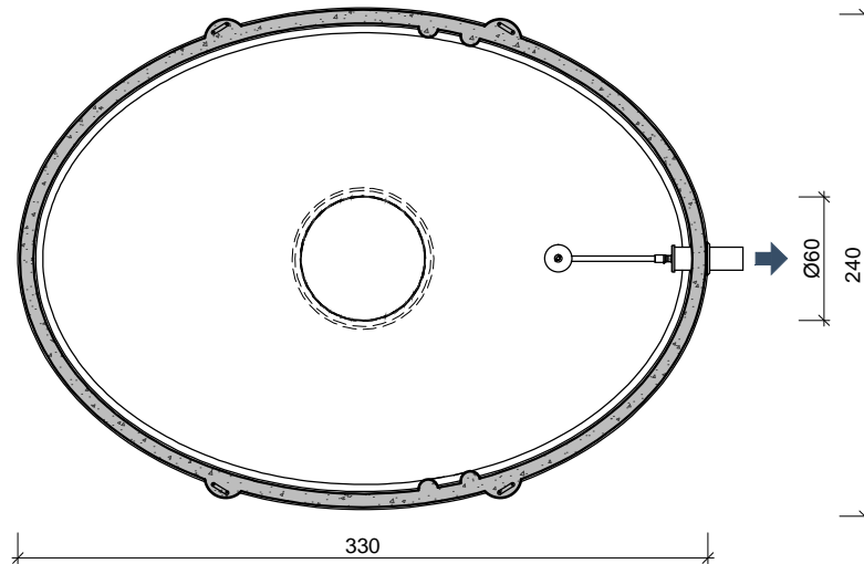
BOVENAANZICHT VUE DE DESSUS
