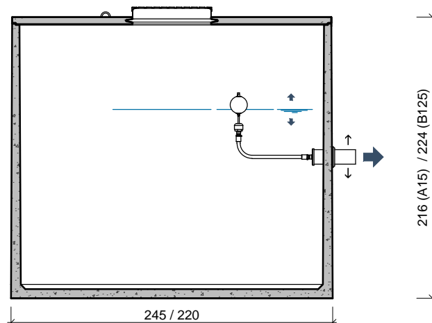
DOORSNEDE COUPE
